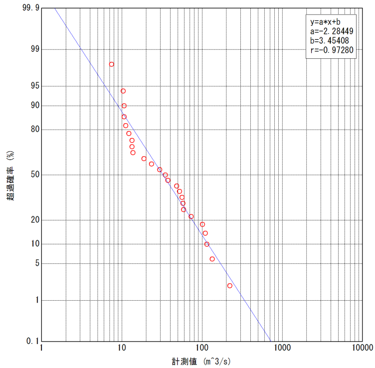
図1 対数正規確率分布のプロット例
